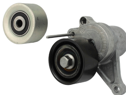
Obrázek 1: Napínací a vodící kladka z kovu
