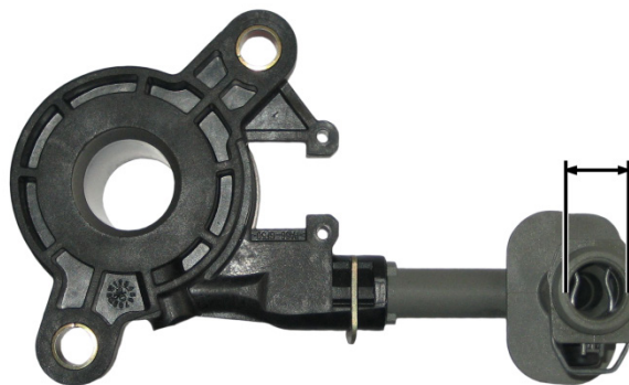
Obr. 2: CSC 3182 600 129 → 3182 654 146 → 3182 654 299 Hydraulický přívod o průměru 13,3 mm
