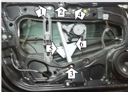
POWER WINDOW LEFT ALZACRISTALLI ELETTTRICO SX
